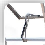
Automatischer Fensteröffner
